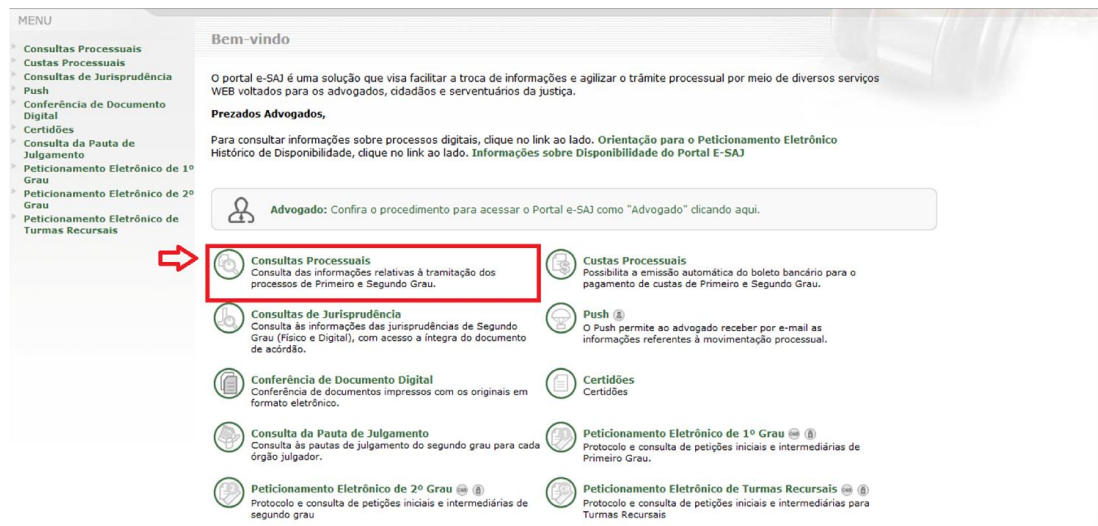
Imagem 2: Consultas Processuais
